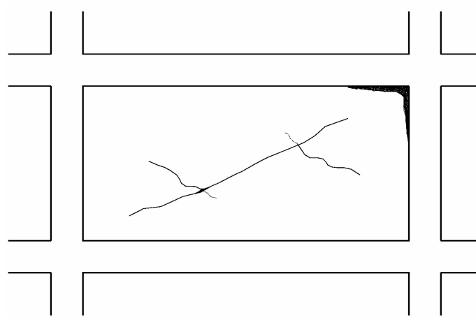
Σ2.2 : Σοβαρή βλάβη τοιχοπλήρωσης, ρωγμές &gt; 5mm
