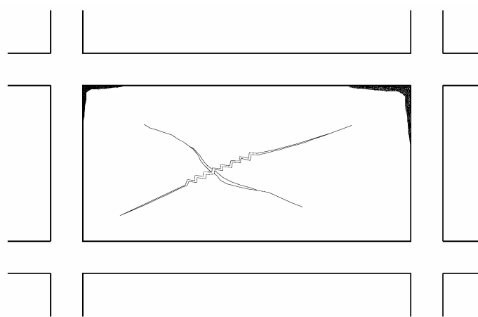
Σ2.3 : Βαριά βλάβη τοιχοπλήρωσης, ρωγμές &gt; 10mm
