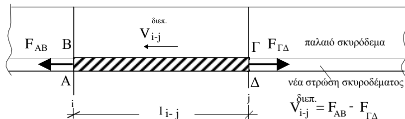
Σχ. Σ8.2: Διατμητική δύναμη στη διεπιφάνεια
