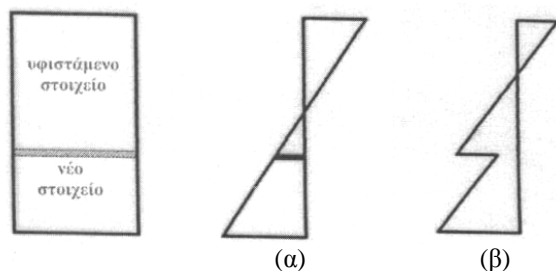
Σχ. Σ8.1: Κατανομή παραμορφώσεων σε καμπτόμενη σύνθετη διατομή :
