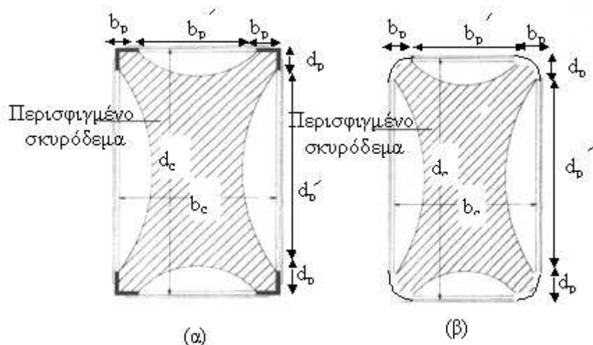
Σχ. Σ6.9 (α) Περίσφιγξη με χαλύβδινο κλωβό (β) Περίσφιγξη με ινωπλισμένα πολυμερή-στρογγύλευση γωνιών, βλ. § 4.4.3.ε
