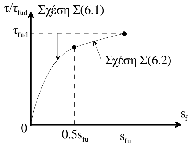
Σχ. Σ6.3: Διάγραμμα διατμητικών τάσεων-σχετικών ολισθήσεων κατά μήκος τραχειάς διεπιφάνειας σκυροδέματος (σηματικό).
