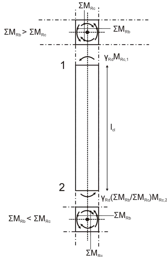
Σχ. Σ.9.1 Ενδεικτικό παράδειγμα καμπτικών αντιστάσεων στα άκρα υποστυλωμάτων για ικανοτικόν υπολογισμόν τέμνουσας δύναμης
