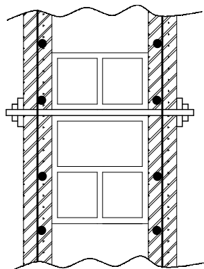
Σχ. Σ8.9: Ενδεικτική τομή εφαρμογής ενίσχυσης υφιστάμενης πλινθοπλήρωσης
